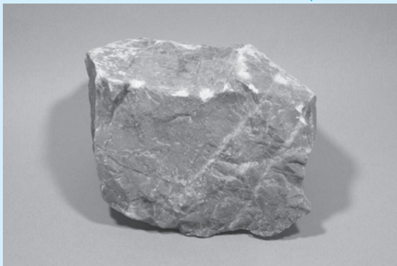
▲石灰岩（豊後大野市資料館蔵）
