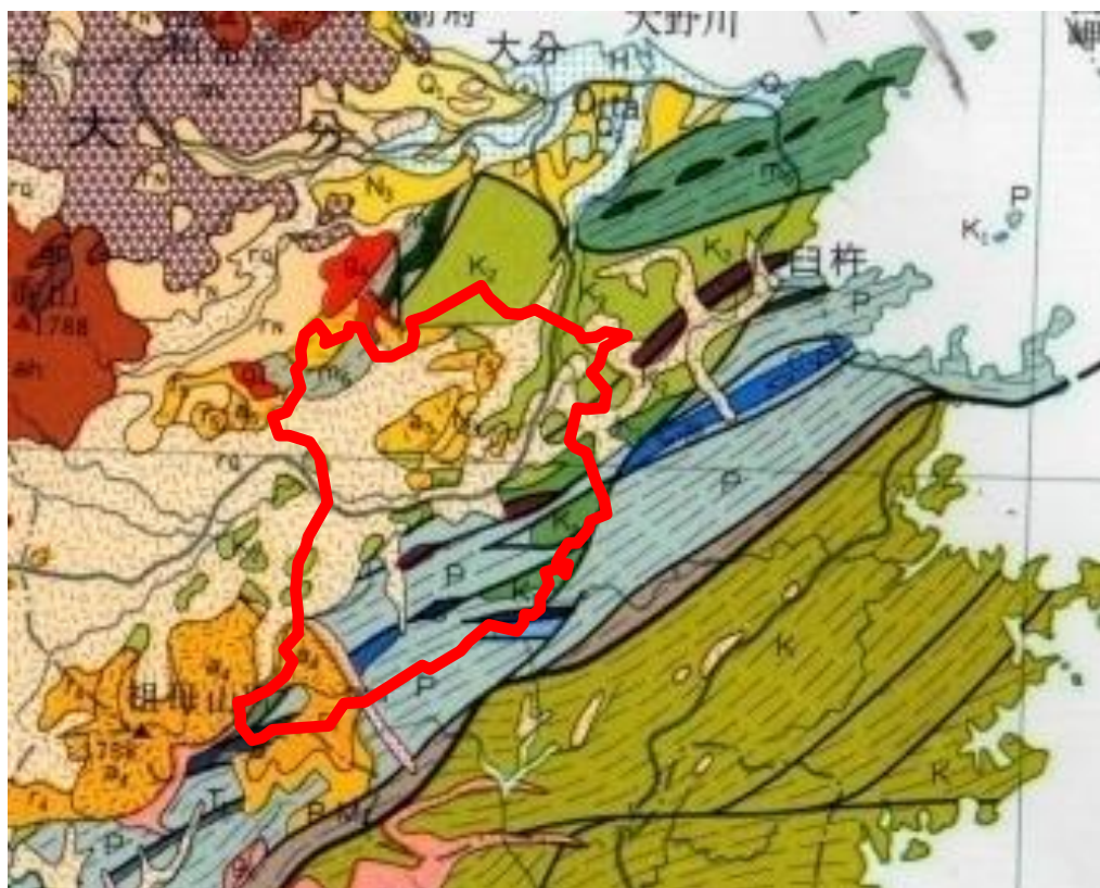
大分県の地質図
