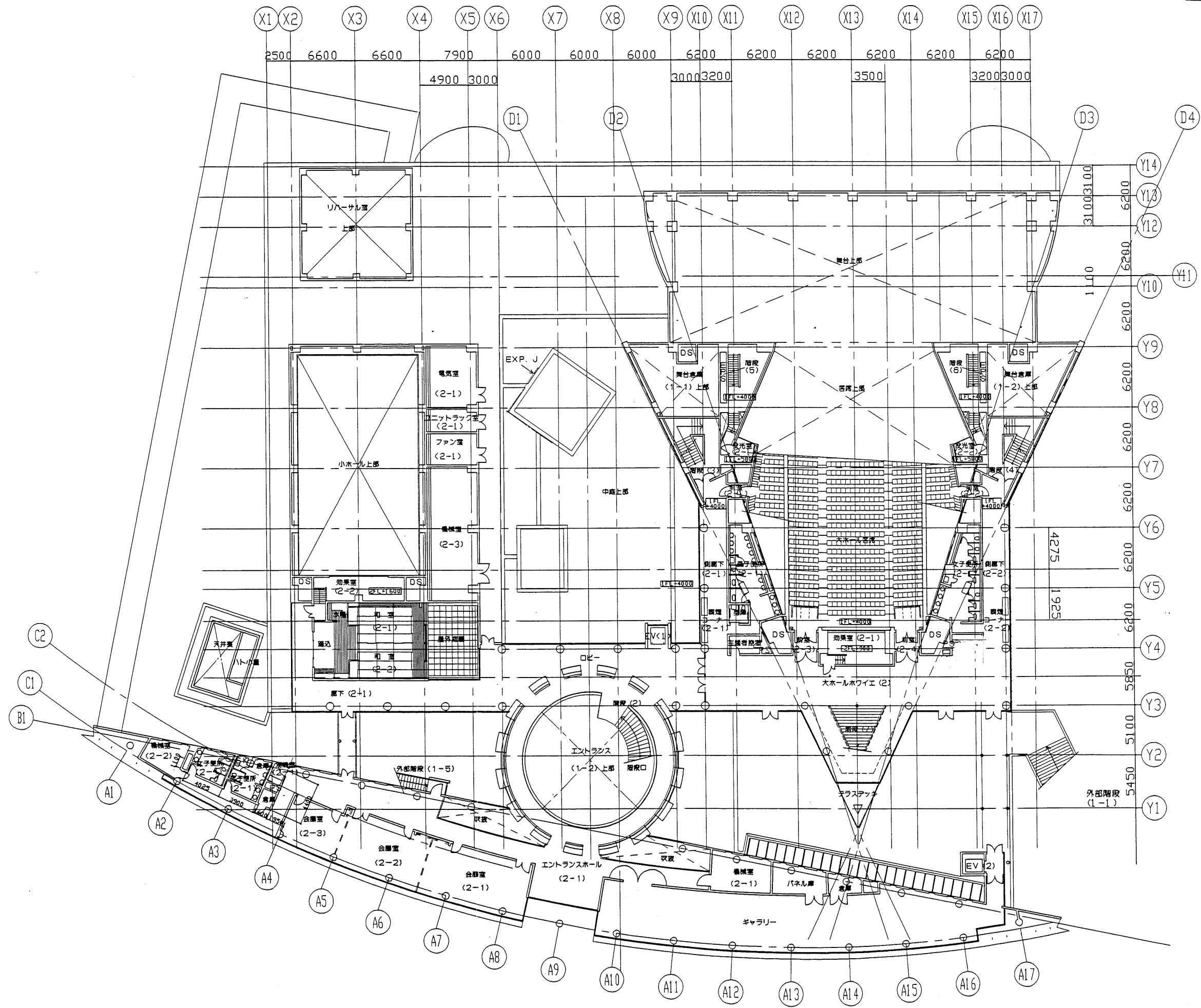
2階平面図
