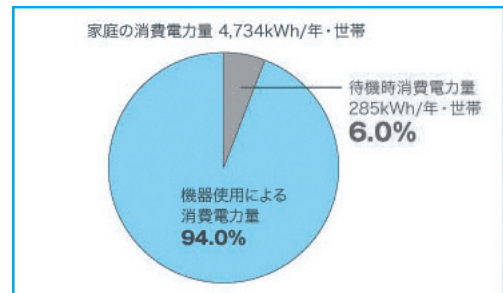
家庭の消費電力量に占める待機時消費電力量の割合
