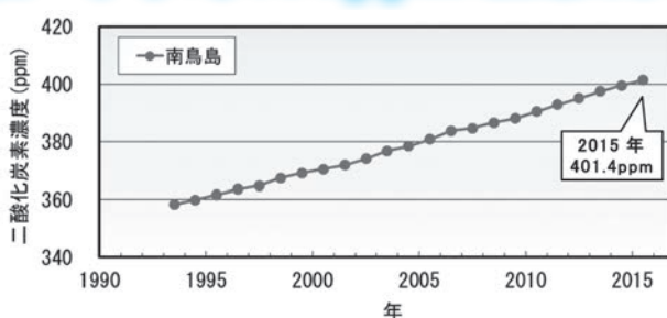
図 南島における大気中二酸化炭素濃度の年平均値の経年変化
